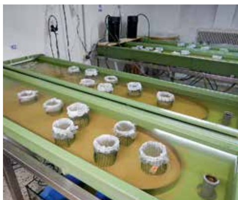
Abbildung 9 Jungmuschel-Hälterungsrinnen als Beispiel für die permanenten Versuche mit alternativen Methoden.
